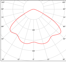
BALK20CY, BALK30CY
