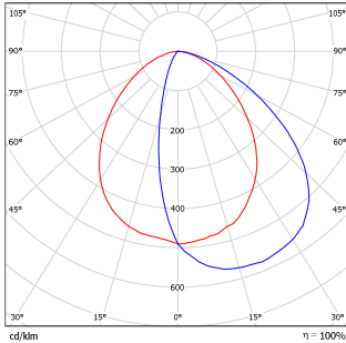
aluevalaisu
