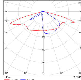
leveät kulkuväylät
