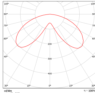
aluevalaisu
