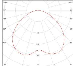
cd/km — C0 - C180 aluevalaisu
